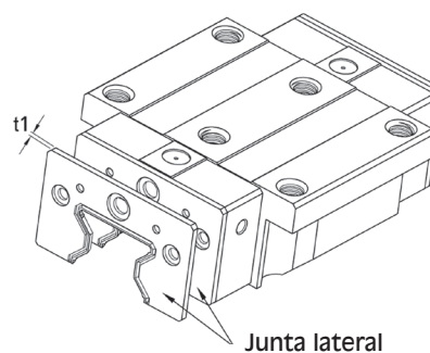
DD: 2 Juntas laterales y Junta inferior
