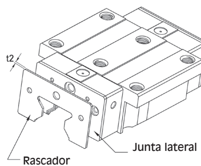
ZZ: Junta lateral, rascador y Junta inferior
